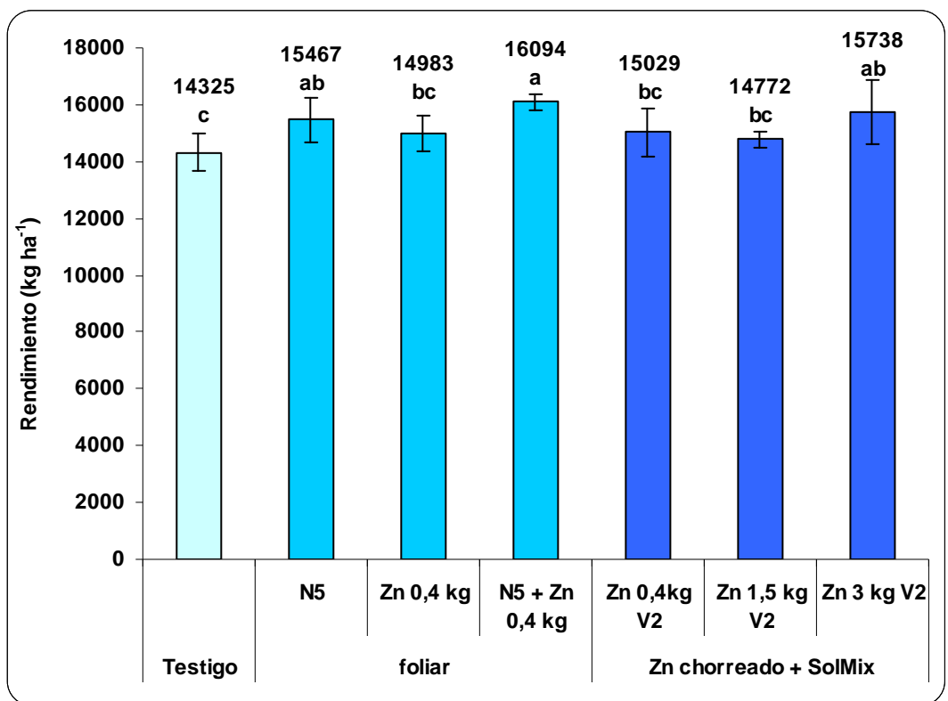
Figura 4: Producción de grano de maíz ( kg\ ha^{-1} ) en tratamientos de fertilización con zinc aplicado al suelo o foliar en combinación con fuentes nitrógeno-azufradas. Letras distintas en las columnas indican diferencias estadísticamente significativas entre tratamientos. Las barras verticales representan la desviación Standard de la media. Pergamino, Campaña 2009/10.
