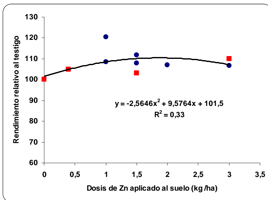
Figura 6: Relación entre los Rendimientos Relativos de maíz ( RR = (\text{Rendimiento Zn en kg ha}^{-1} / \text{Rendimiento testigo}) \times 100 ) y la dosis de Zn aplicada al suelo, junto a soluciones fertilizantes que contienen NS.
